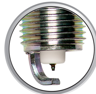
ELECTRODO CENTRAL CON PUNTA DE PLATINO
